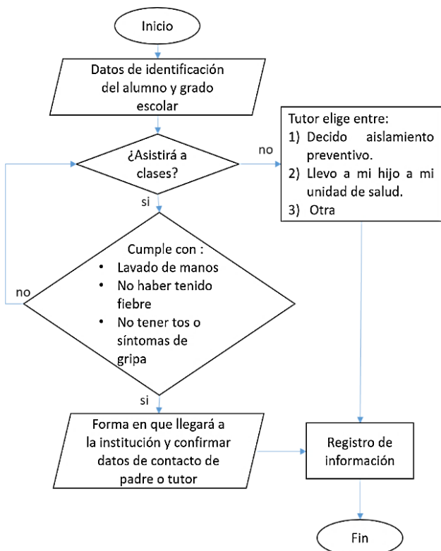
Fig. 2 Esquema de funcionamiento de filtro sanitario virtual para el Sistema Educativo Adventista.
